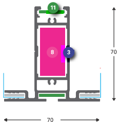
3 131726/28 Multiframe® 70 T-povezovalni profil (horizontalni)
